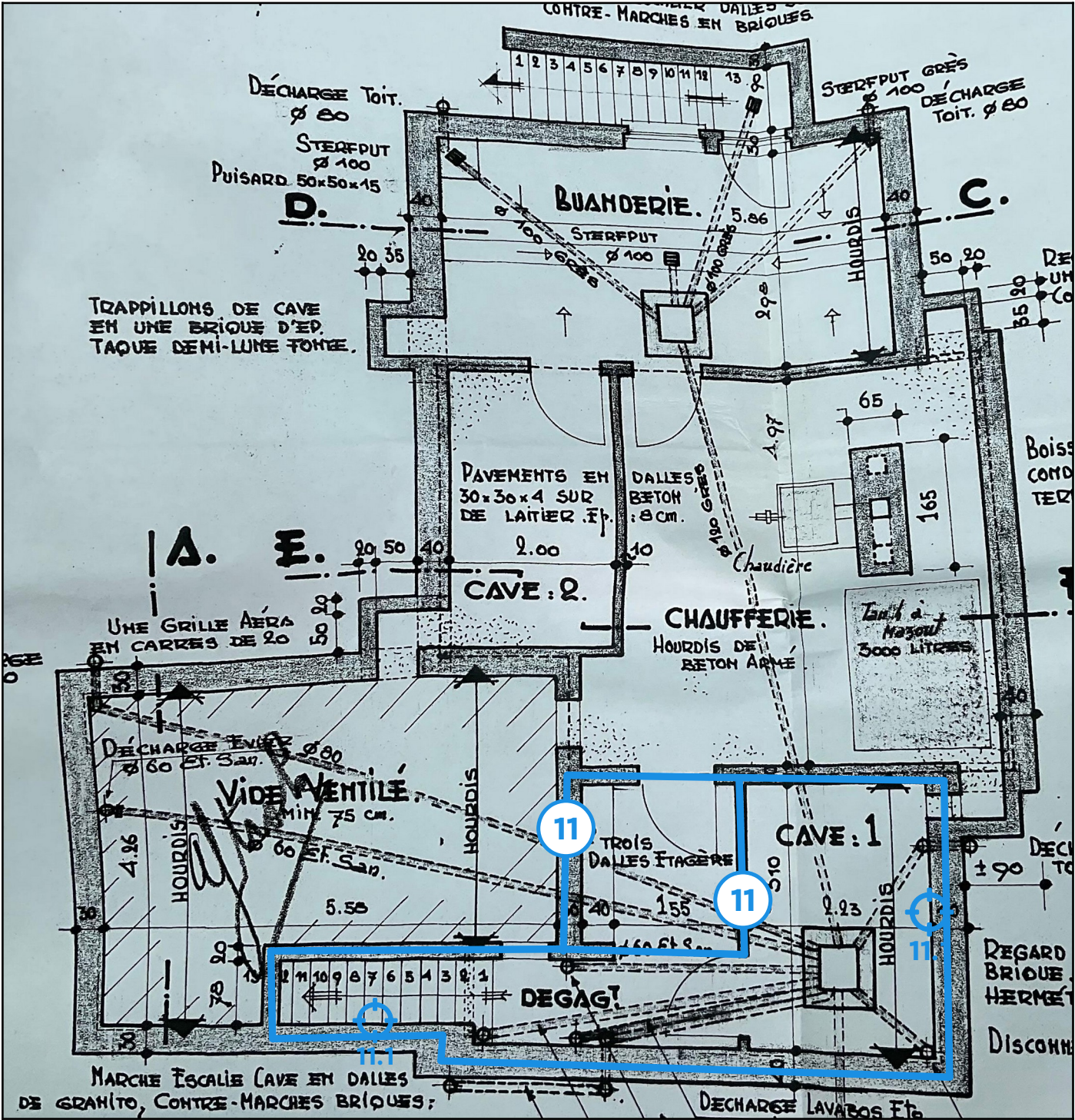
Legende van plan 1.2: Kelder (wandpleister)
